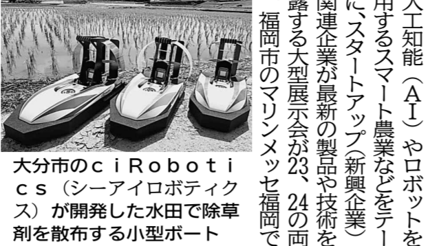
大分市のCiRobotics(シーアイロボティクス)が開発した水田で除草剤を散布する小型ロボット
